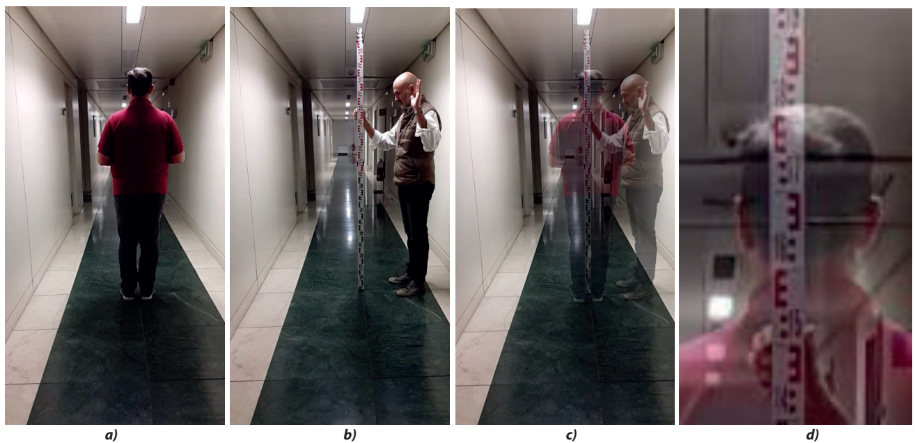
Figura 2 - Esempio di impiego della stadia metrica. a) immagine originale del soggetto da misurare; b) stadia metrica posta nella stessa posizione del soggetto di interesse; c) sovrapposizione delle immagini in a) e b); d) particolare della sovrapposizione.
